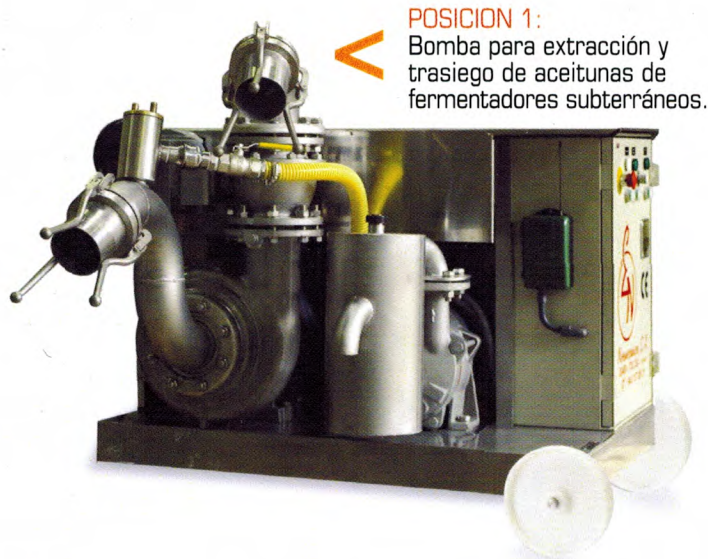
Bomba para extracción y trasiego de aceitunas de fermentadores subterráneos. Aspiración mediante válvula de cebado manual.
