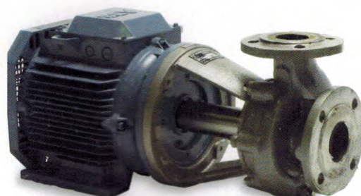
Bomba autoaspirante para retorno de salmuera con cebado por bomba de vacío.
